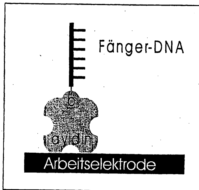
Abbildung 18: Immobilisierung der einzelsträngigen DNA als analyterkennendes Element über Avidin auf der Arbeitselektrode
